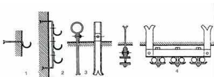
Сл. 39. Кабловска обумица: 1 – једнострука отворена, 2 – вишеструка отворена, 3 – једнострука затворена, 4 – вишеструка полуотворена
