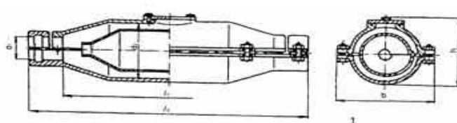
Сл. 37. Права оклопна спојница са унутрашњом оловном, за радни напон до 1 kV: 1 – цртеж спојнице у две пројекције; 2 – спојница са прибором за монтажу (везна жица, уље за уземљење), изолациона трава, импрегнирани папир, азбестна трака, јутана трака, паста за лемљење, стерион и маса за ваљање, унутрашње и спољне заштитне спојнице
